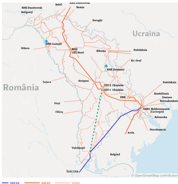
Fig. 11. Noua linie electrică de 400 kV Vulcănești–Chișinău (cu verde). 95
